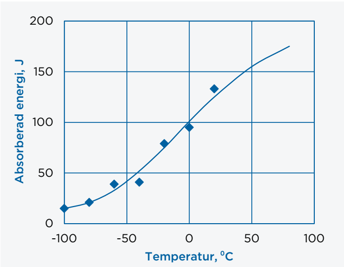
Omslagskurvan från Charpy-V provning av SS-EN 4162 (Outokumpu LDX 2101*), ett duplex rostfritt stål. Omslagstemperaturen, t.ex. temperaturen då den absorberade energin är 27 J, är i detta fall ca -70°C. Mätvärden för absorberad energi är tagna ifrån ett bidrag av H. Sieurin, E. Westin, M. Liljas och R. Sandström till konferensen "Duplex 2007" som organiserades av Associazione Italiana di Metallurgia, Grado, Italien (2007).
