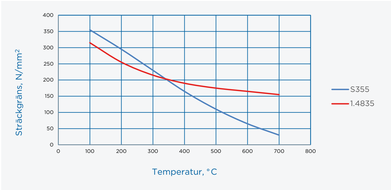
Sträckgränsens beroende av temperatur för konstruktionsstålet S355 och det värmebeständiga austenitiska rostfria stålet SS-EN 1.4835 (Outokumpu 253 MA®).
