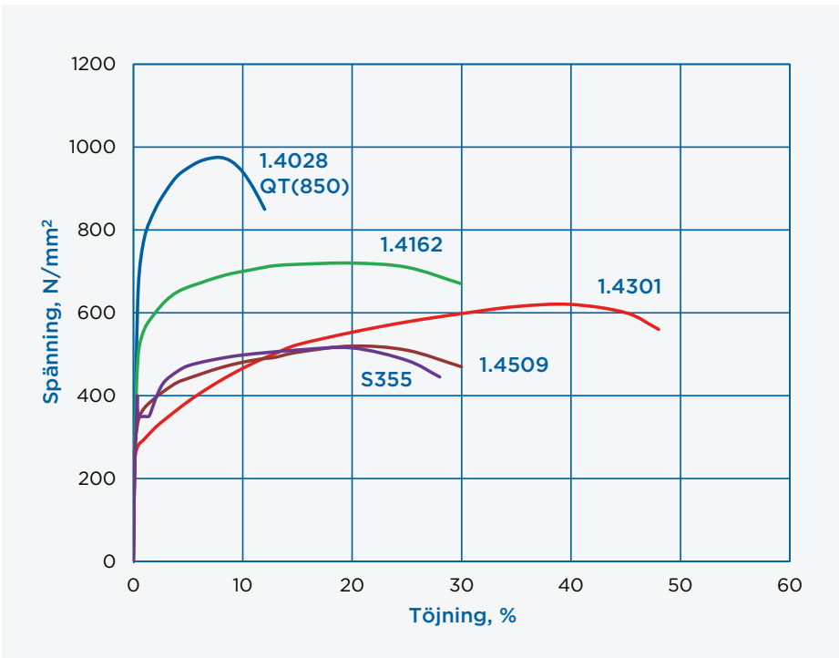
Jämförelse av spännings-töjningskurvor för olika typer av rostfritt stål samt ett konstruktionsstål, S355 (1.4028 martensitiskt, 1.4162 duplext, 1.4301 austenitiskt och 1.4509 ferritiskt)
