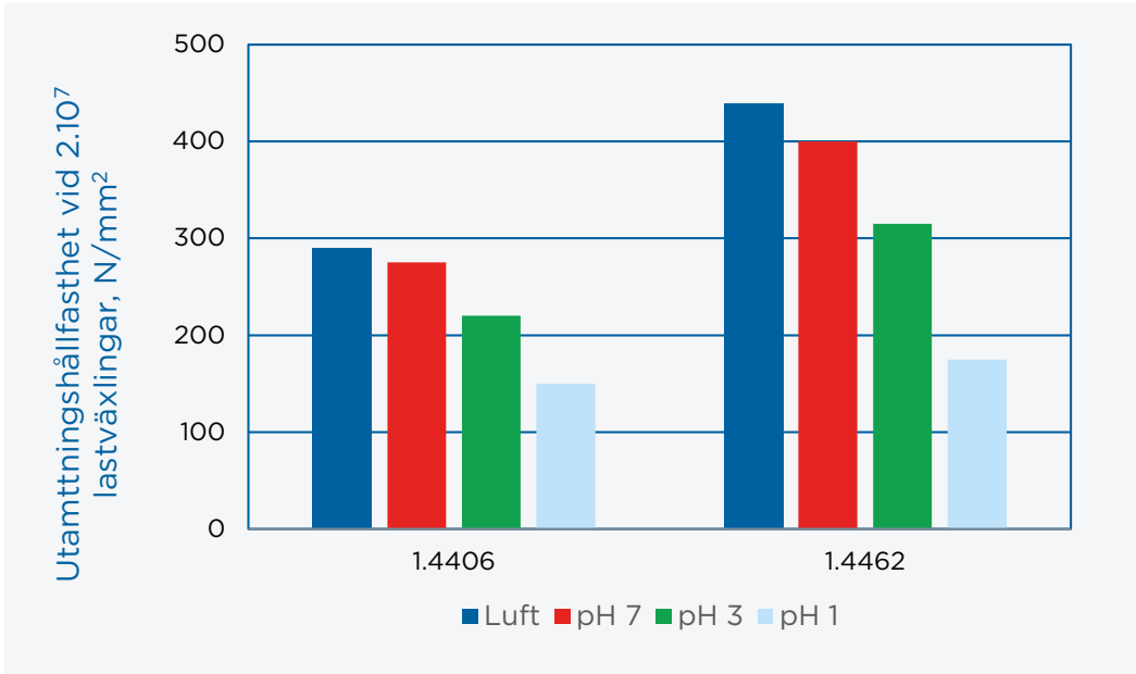
Inverkan av miljö på utmattningshållfasthet för ett austenitiskt och ett duplext stål testade i roterande böjprovning vid 40°C i luft och 3% saltlösningar av olika surhetsgrad. Diagrammet är reproducerat från Outokumpus publikation "Handbook of Stainless Steel".
