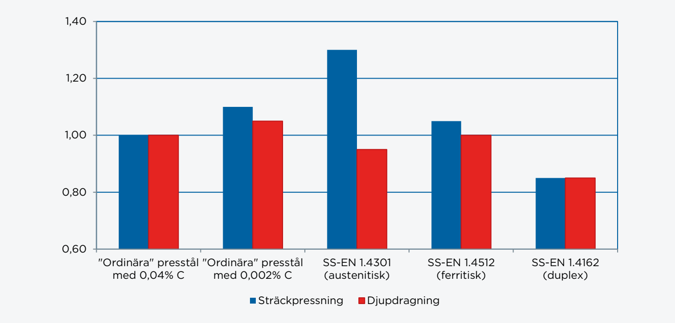
Ungefärlig jämförelse av formbarhet av olika typer av rostfria stål i förhållande till ett ordinärt presstål med 0,04 % C. Avser samma plåttjocklek men eftersom tjockleken ofta kan minskas för duplexa stål (tack vara den högre hållfastheten) kommer formbarheten då att förbättras i förhållande till de andra.
