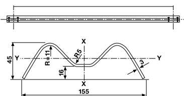
Navföljare rak I_y = 8,2 \times 10 \text{ mm}^2 W_y = 3,0 \times 10 \text{ mm}^2 L=4,3 m, art.nr: 82066 L=2,7 m, art.nr: 72835 L=2,3 m, art.nr: 98923
