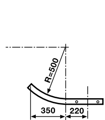
Ändstycke Halvbockat Art.nr: 179094
