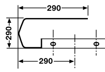
Ändstycke Rakt för enkelräcke Art.nr: 179101
