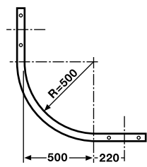
Ändstycke 90° R = 500 mm Art.nr: 179092
