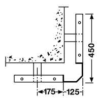
Kort ändstycke 90° För montage på vägg/pelare Art.nr: 179095 Innehörn Art.nr: 179102
