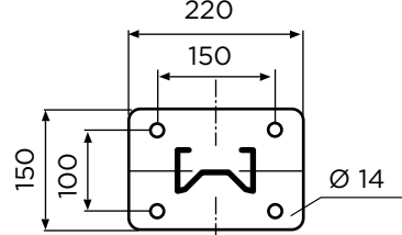
Sigma stolpe med fotplåt PL.8x150x220 Art.nr: 179105
