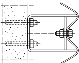
Väggmonterat skyddsräcke
