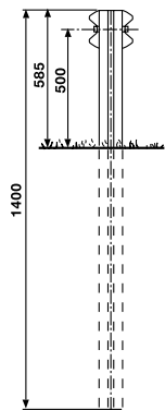
Mini-W skyddsräcke Dubbelt
