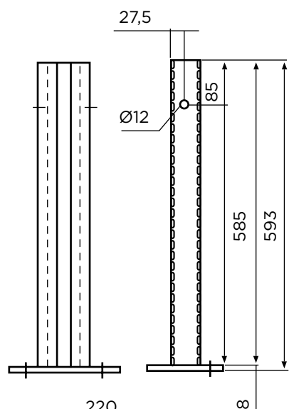
Ändstycke Halvbockat Art.nr: 179094
