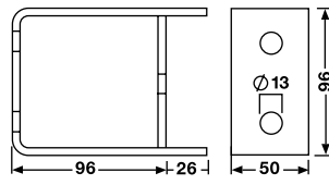
Distansfäste För vägg Art.nr: 179097
