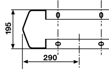
Ändstycke Rakt för dubbelräcke Art.nr: 179103
