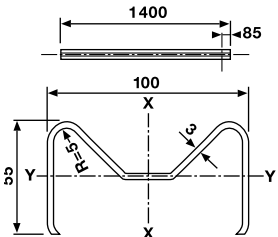
Tung Sigma stolpe Godstjocklek 4 mm Art.nr: 179099
